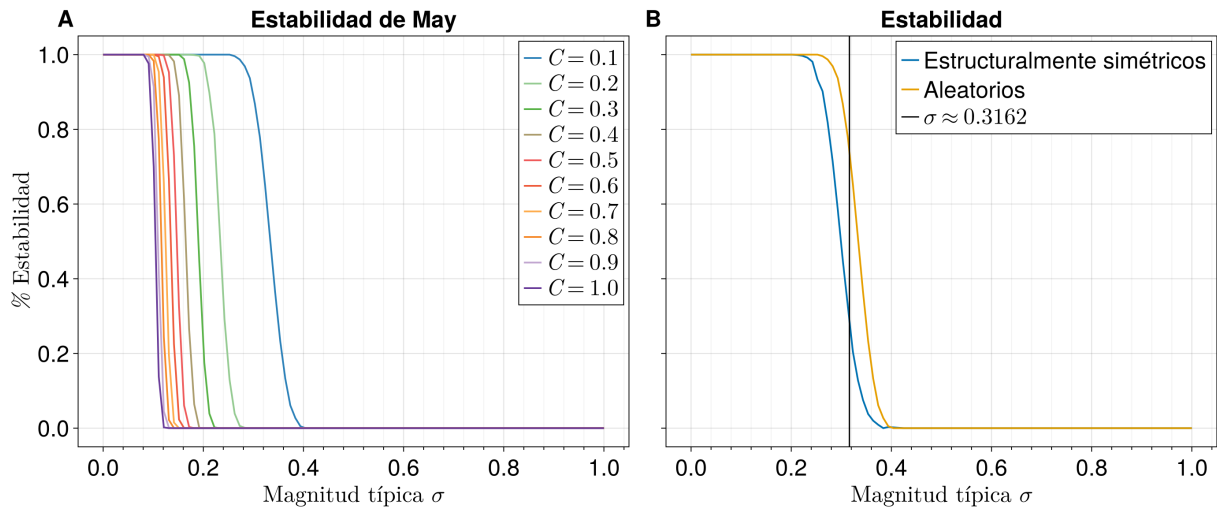
Figura 1.11: Transición dinámica en función de \sigma (A) Se consideran sistemas de May aleatorios con 3000 simulaciones por cada configuración. (B) Caso particular para C = 0.1 ; se consideran las diferencias entre sistemas de soporte simétrico y puramente aleatorios.
