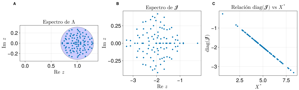
Figura 3.7: Se muestra una realización de un estado coexistente con soporte dirigido para los parámetros N = 100 , p = 0.1 y \sigma = 0.1 . (A) Espectro de \Lambda asociada. (B) Espectro de la Jacobiana asociada. (C) Relación lineal \text{diag}(\mathcal{J}) vs X^* .
