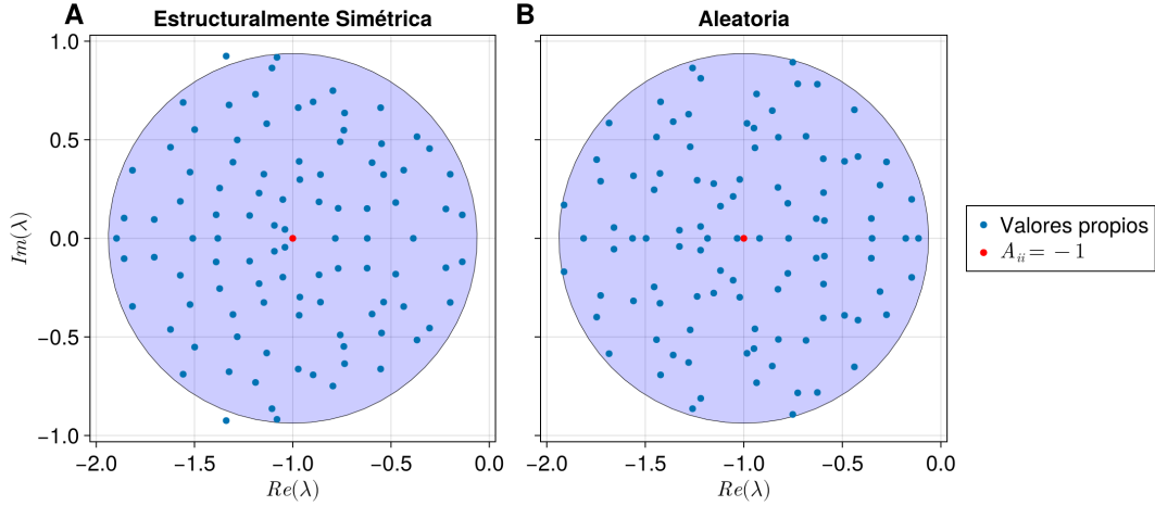
Figura 1.6: Distribución de valores propios en sistemas de May con soporte simétrico y puramente aleatorios. En ambos casos se consideró N = 100 , magnitud típica \sigma = 0.2 , para una conectividad C = \frac{1}{\sigma^2 N} - 0.03 .
