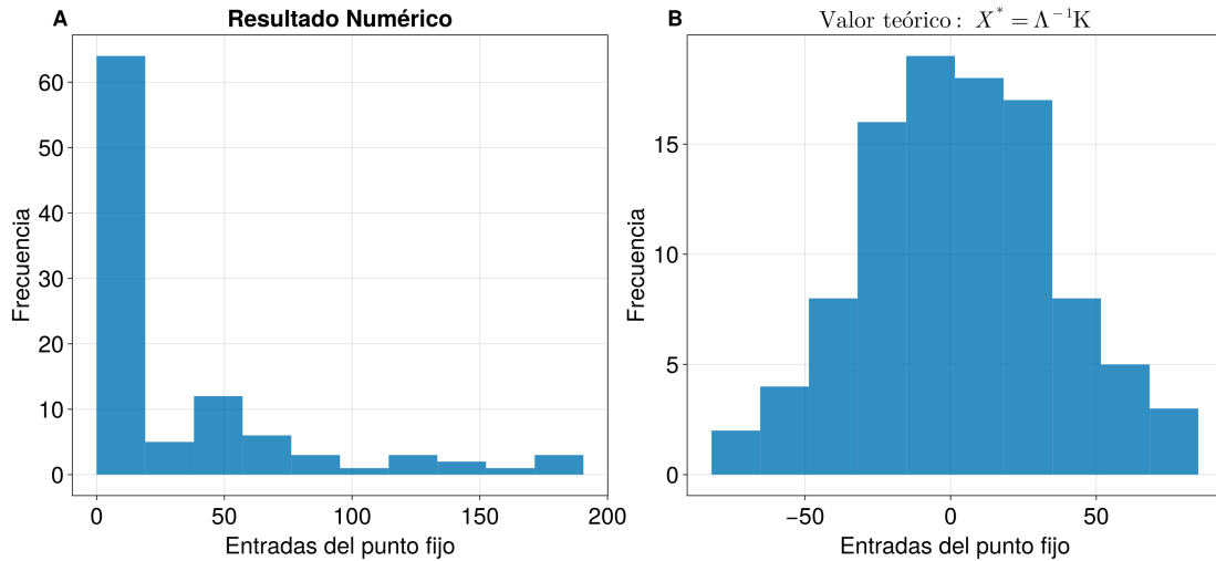
Figura 3.6: Distribución del punto fijo para una realización con p = 0.5 y \sigma = 0.2 .
