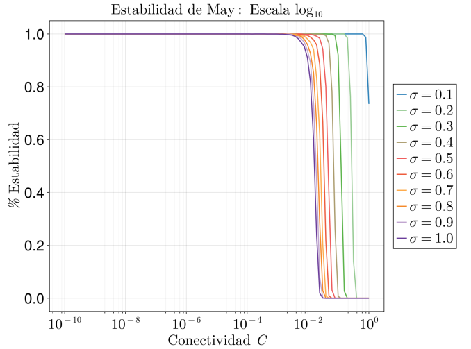
Figura 1.9: Transición dinámica en sistemas de May aleatorios en función de C en escala \log_{10} .
