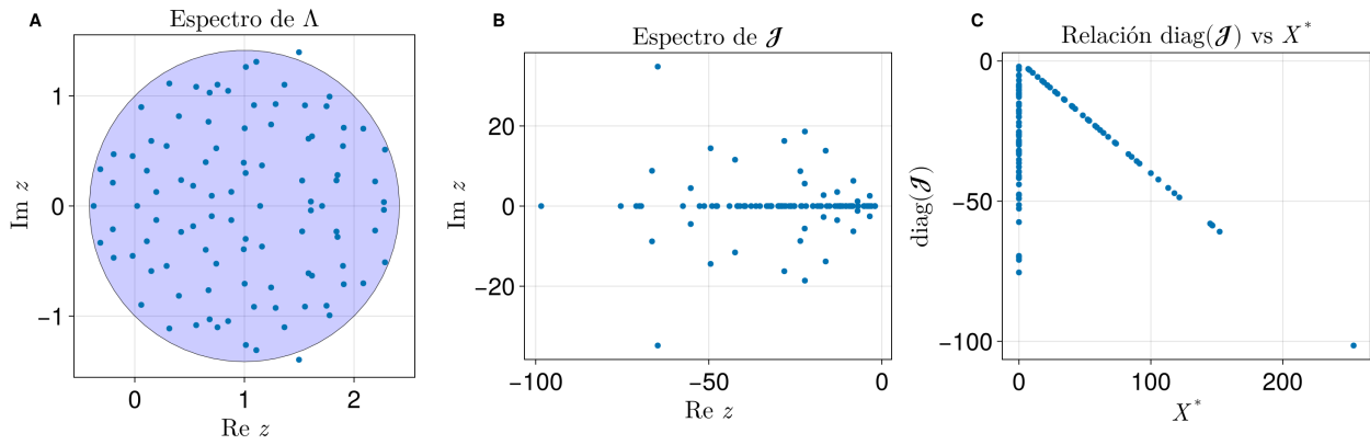
Figura 3.8: Se muestra una realización de un estado parcialmente factible con soporte dirigido para los parámetros N = 100 , p = 0.5 y \sigma = 0.2 . (A) Espectro de \Lambda asociada. (B) Espectro de la Jacobiana asociada. (C) Relación lineal \text{diag}(\mathcal{J}) vs X^* .
