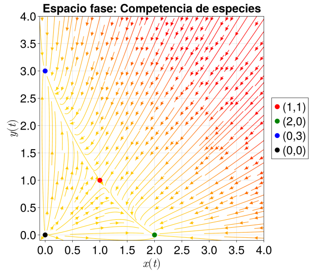
Figura 1.3: Campo vectorial de las soluciones del sistema (1.3) de dos especies.
