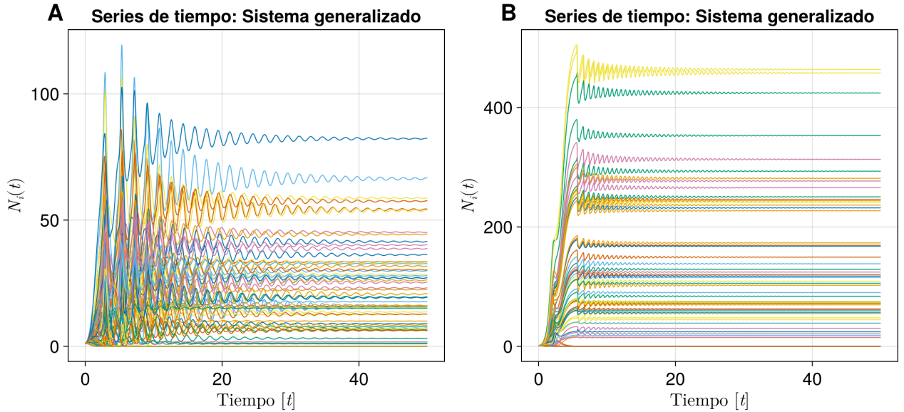
Figura 3.2: Series de tiempo del sistema Lotka–Volterra generalizado. (A) Se consideran los parámetros p = 0.35 , \sigma = 0.2 y N = 100 para \Lambda . (B) Se consideran los parámetros p = 0.5 , \sigma = 0.2 y N = 100 para \Lambda .
