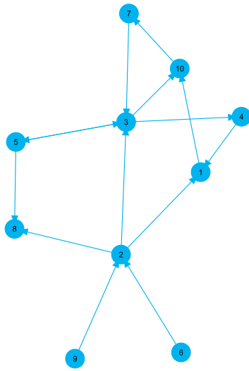
Figura 1.2: Red dirigida de 10 nodos.
