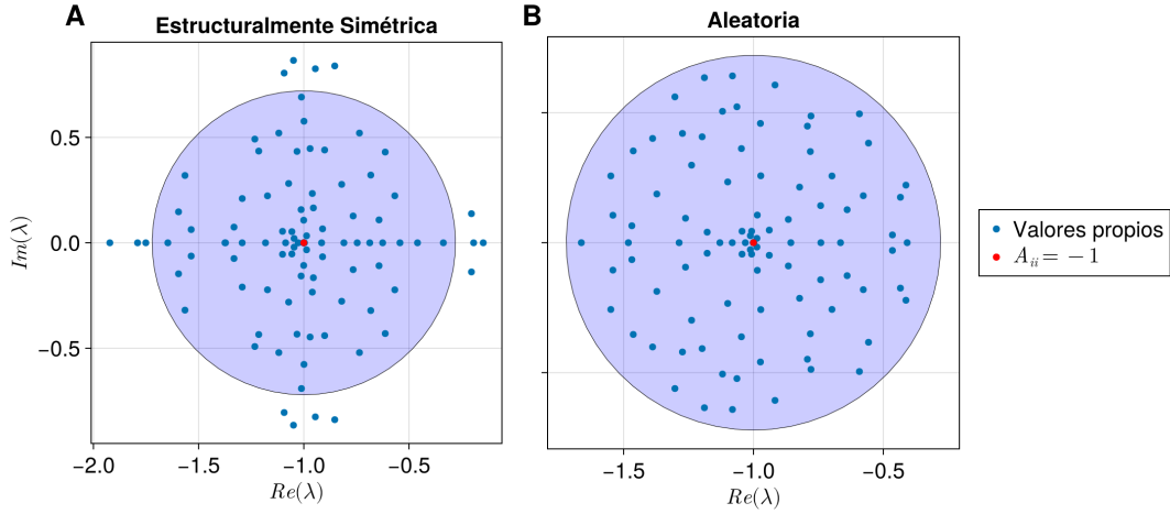
Figura 1.7: Distribución de valores propios en sistemas de May con soporte simétrico y puramente aleatorios. En ambos casos se consideró N = 100 , magnitud típica \sigma = 0.4 , para una conectividad C = \frac{1}{\sigma^2 N} - 0.03 .
