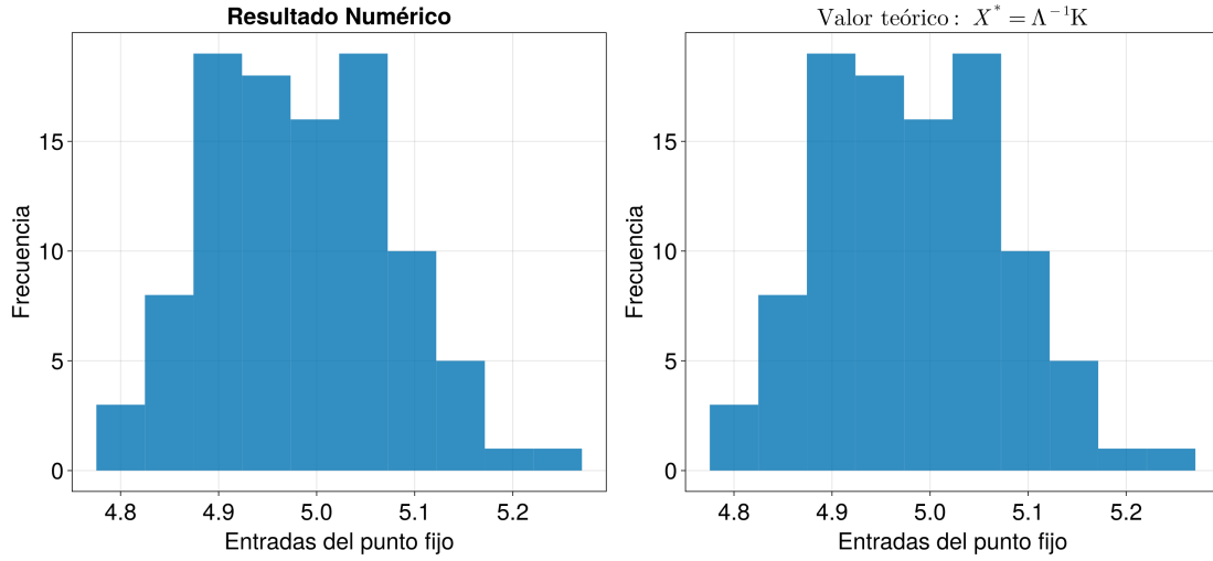
Figura 3.4: Distribución del punto fijo para una realización con p = 0.5 y \sigma = 0.003 .
