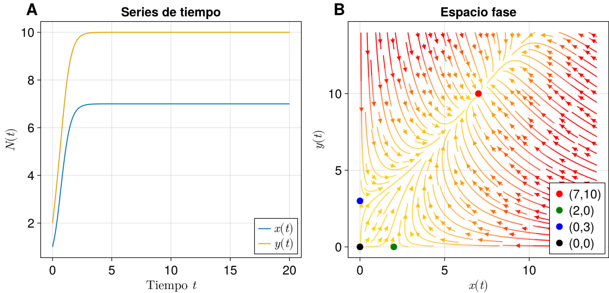
Figura 1.4: Sistema de Lotka–Volterra con interacciones de cooperación dados por las ecuaciones (1.6). Tasas de crecimiento y capacidades de carga: r_x = K_x = 2 y r_y = K_y = 3 . (A) Series de tiempo del sistema para las especies x(t) y y(t) bajo la condición inicial (1, 2) . (B) Espacio fase del sistema con sus puntos fijos asociados, se muestra solamente un único punto fijo estable.
