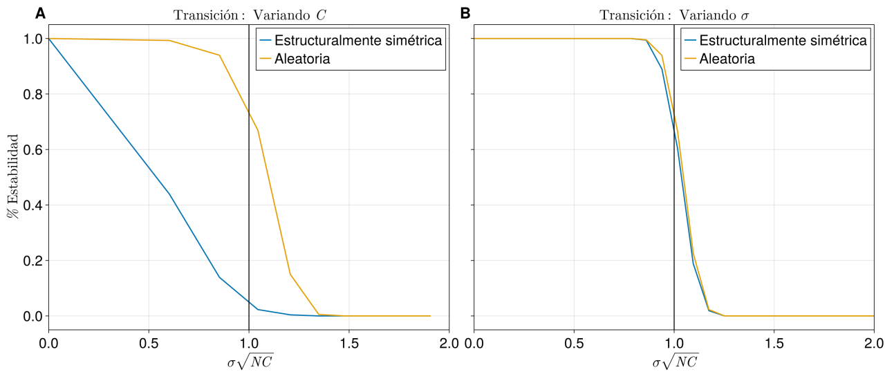
Figura 1.14: Re-escalamiento del eje x para visualizar las transiciones de la conectividad C y la fuerza promedio de las interacciones \sigma . Para este caso particular se escogió \sigma = C = 0.6 . Se consideran matrices de puramente aleatorias y estructuralmente simétricas.
