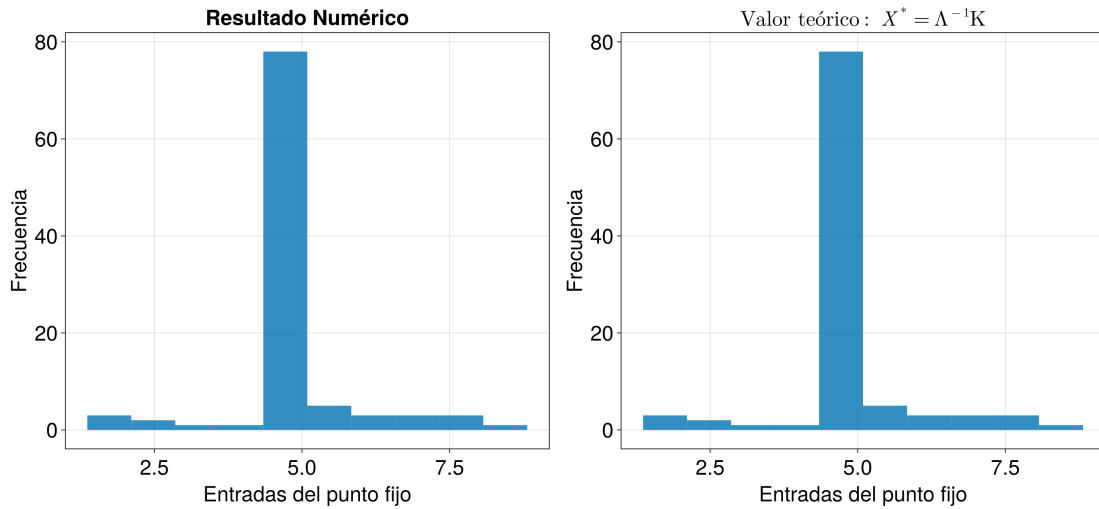
Figura 3.5: Distribución del punto fijo para una realización con p = 0.003 y \sigma = 0.5 .
