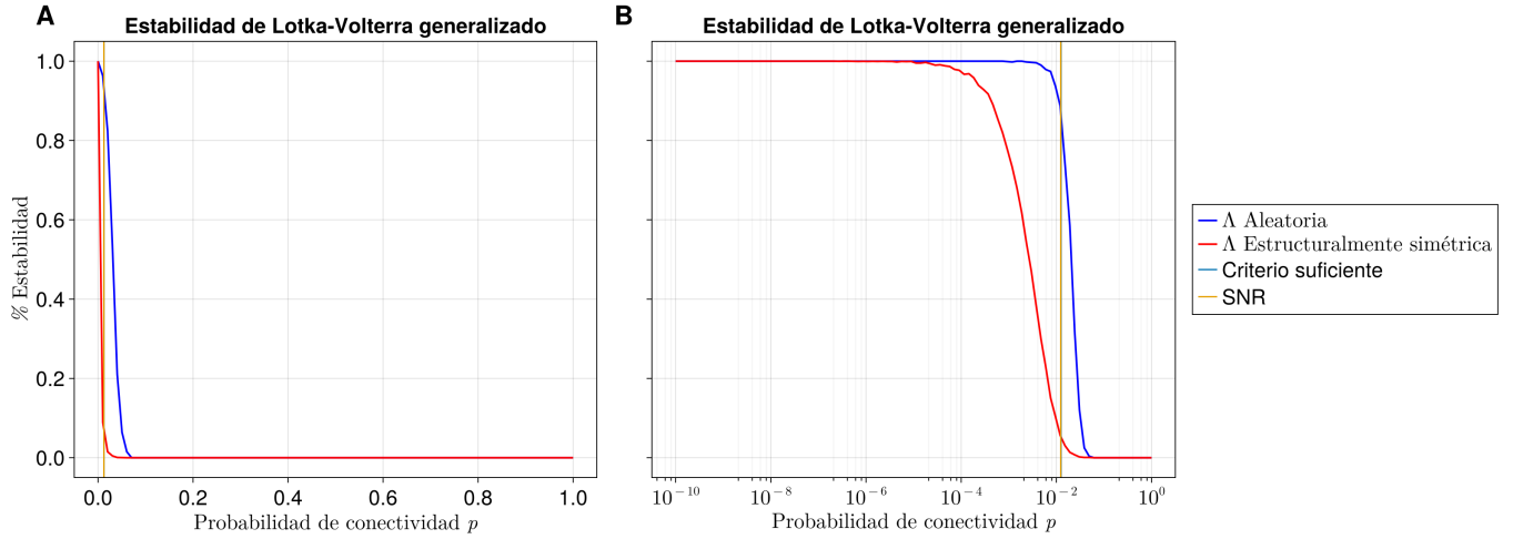
Figura 4.16: Transición dinámica para el caso \sigma = 1.0 considerando \kappa = 0.9 . (A) Escala lineal. (B) Escala logarítmica.
