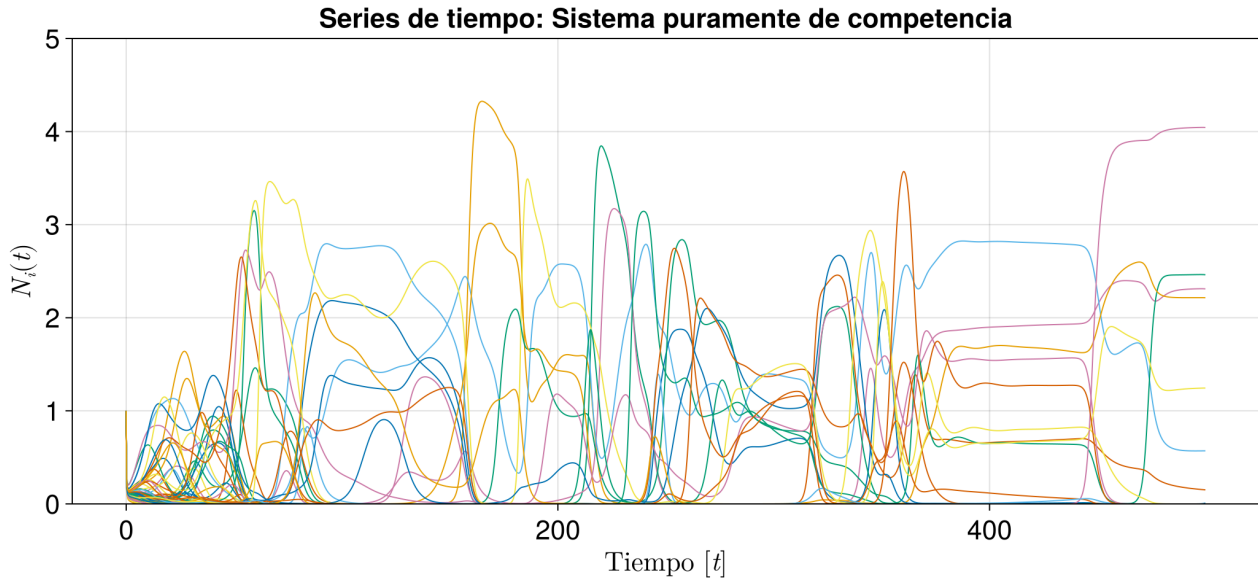
Figura 3.1: Series de tiempo para el sistema de competencia de N = 100 especies. Se emplea una matriz \Lambda cuyas entradas provienen de una distribución uniforme del intervalo [0, 1] para p = 1.0 . Las especies quedan acotadas por su capacidad de carga K = 5 .
