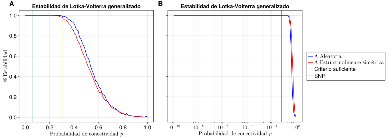
Figura 4.15: Transición dinámica para \sigma = 0.2 considerando \kappa = 0.9 . (A) Escala lineal. (B) Escala logarítmica.
