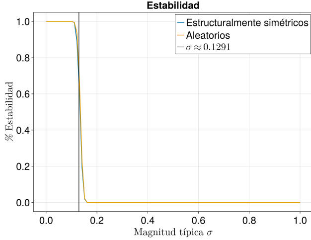
Figura 1.12: Variación de la transición entre sistemas estructuralmente simétricos y puramente aleatorios. Se considera el valor de la conectividad C = 0.6 .
