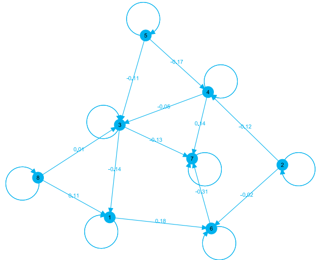
Figura 2.1: Red de interacciones ponderada de 8 nodos con topología de red aleatoria dirigida p = 0.15 y una matriz aleatoria con \mu = 0 y \sigma = 0.2 .
