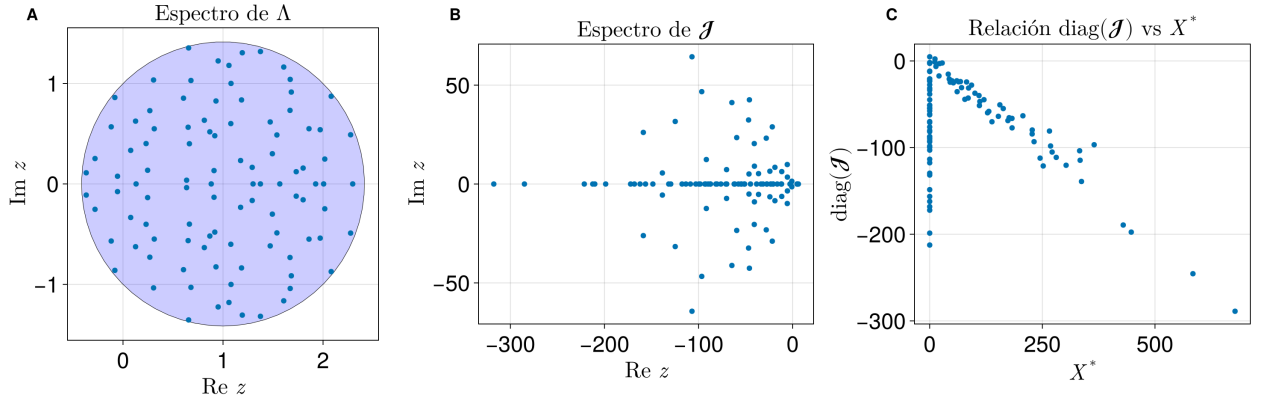
Figura 3.10: Se muestra una realización de \Lambda con soporte estructuralmente simétrico de un estado parcialmente factible para los parámetros N = 100 , p = 0.5 y \sigma = 0.2 . (A) Espectro de \Lambda asociada. (B) Espectro de la Jacobiana asociada. (C) Relación lineal \text{diag}(\mathcal{J}) vs X^* .
