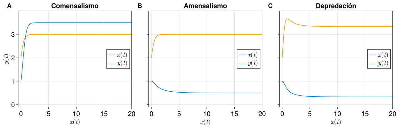
Figura 1.5: Series de tiempo para las interacciones comensalismo, amensalismo y depredación modificando el sistema (1.6). (A) Para el comensalismo se definió \alpha_{21} = 0 y \alpha_{12} = -\frac{1}{2} . (B) Para el amensalismo se consideró \alpha_{21} = 0 y \alpha_{12} = \frac{1}{2} (C) Para la depredación se consideró \alpha_{21} = -1 y \alpha_{12} = \frac{1}{2} .
