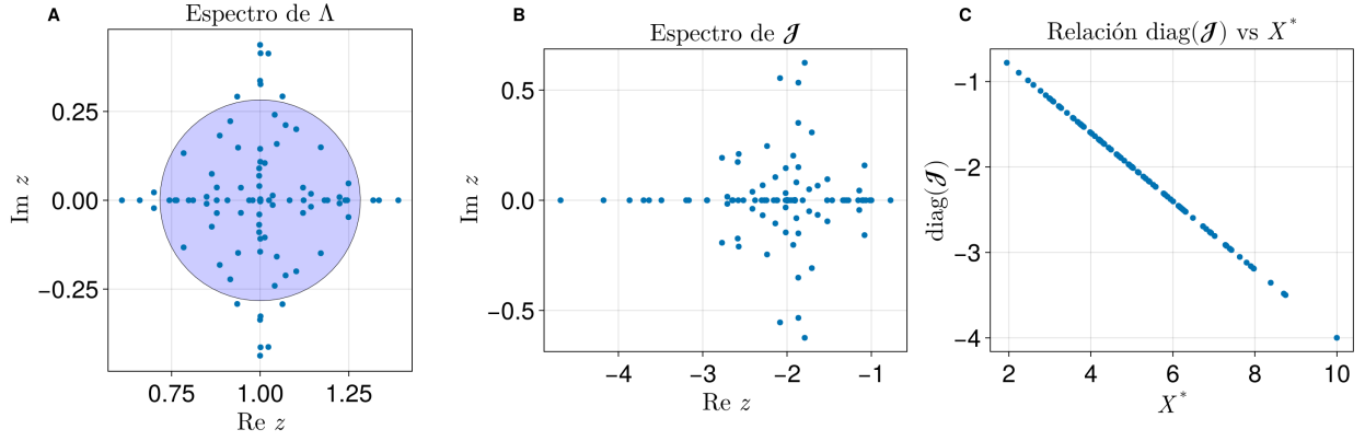
Figura 3.9: Se muestra una realización de \Lambda con soporte estructuralmente simétrico de un estado coexistente para los parámetros N = 100 , p = 0.02 y \sigma = 0.2 . (A) Espectro de \Lambda asociada. (B) Espectro de la Jacobiana asociada. (C) Relación lineal \text{diag}(\mathcal{J}) vs X^* .
