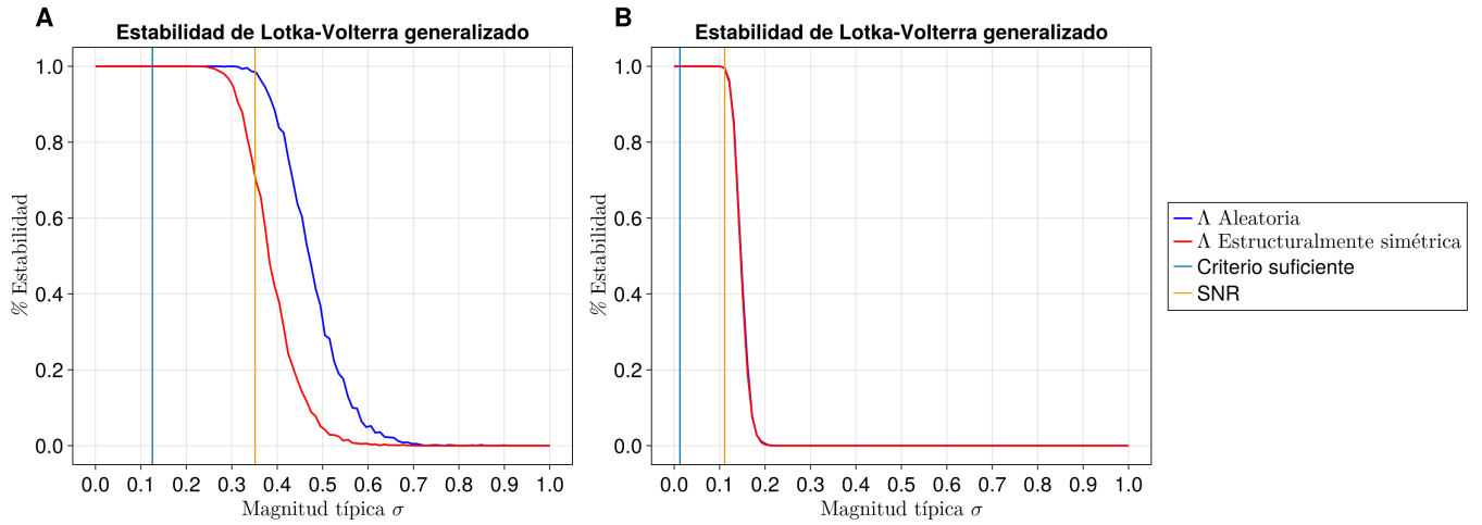
Figura 4.17: Transiciones dinámicas en función de \sigma considerando \kappa = 0.9 . (A) Caso particular para p = 0.1 . (B) Caso particular para p = 1.0 .
