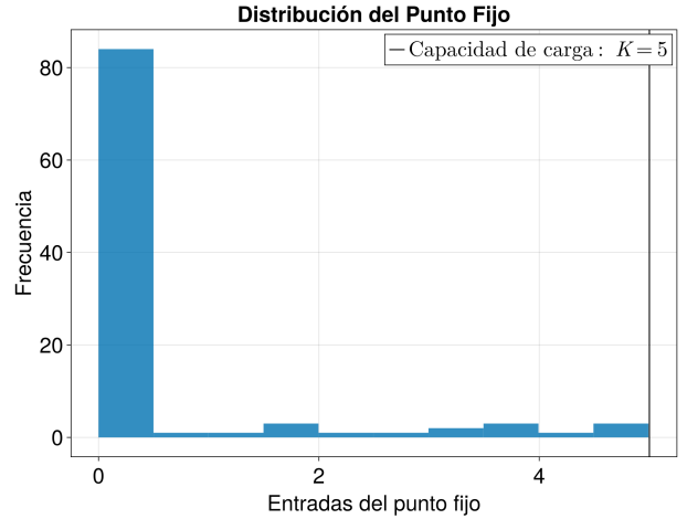
Figura 3.3: Distribución de X^* para sistema de competencia de especies, escogiendo p = 0.5 y considerando una distribución uniforme en los pesos de las interacciones.
