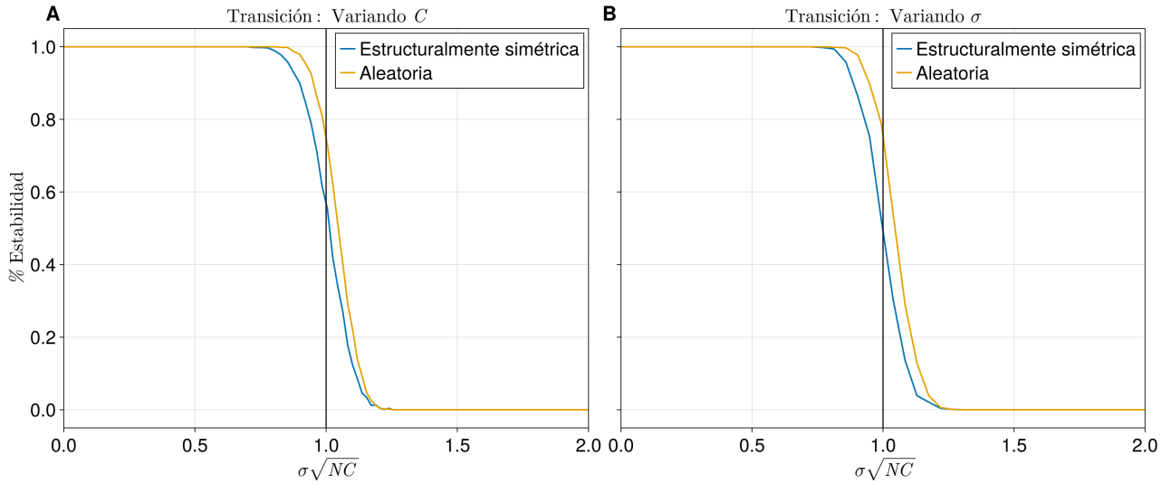
Figura 1.13: Re-escalamiento del eje x para visualizar las transiciones de la conectividad C y magnitud típica de las interacciones \sigma . Para este caso particular se escogió \sigma = C = 0.2 .
