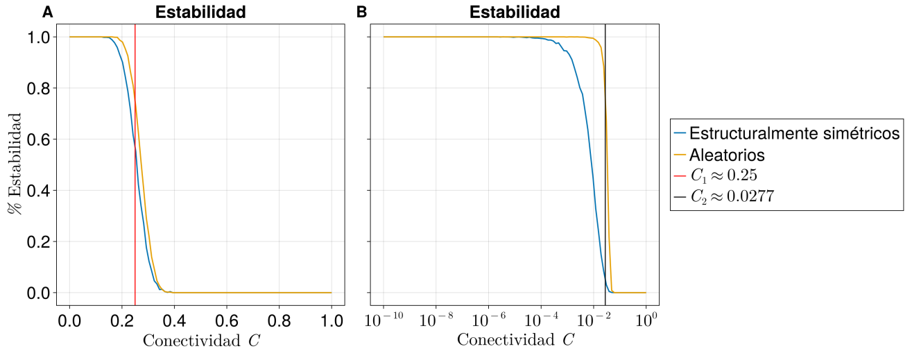
Figura 1.10: Transición de May puramente aleatoria vs estructuralmente simétrica. (A) Se considera para \sigma = 0.2 (B) Se considera para \sigma = 0.6 .
