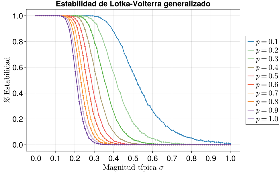
Figura 4.10: Transición dinámica del sistema de Lotka–Volterra generalizado estructuralmente simétrico en función de la fuerza de interacción para N = 50 .
