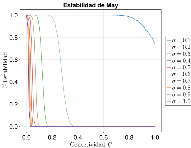
Figura 1.8: Transición dinámica en sistemas de May aleatorios en función de C . Para cada configuración se generan 3000 simulaciones independientes.
